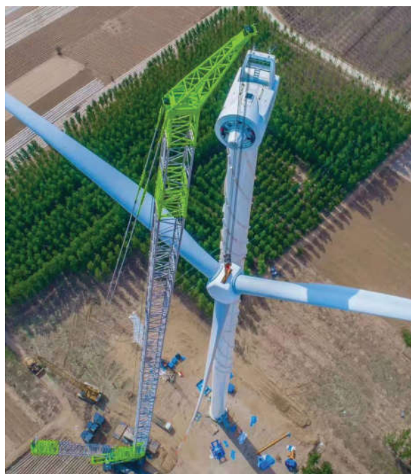
ZCC9800 800T CRAWLER CRANE -CẦN CẦU 800 TẤN ZCC9800
